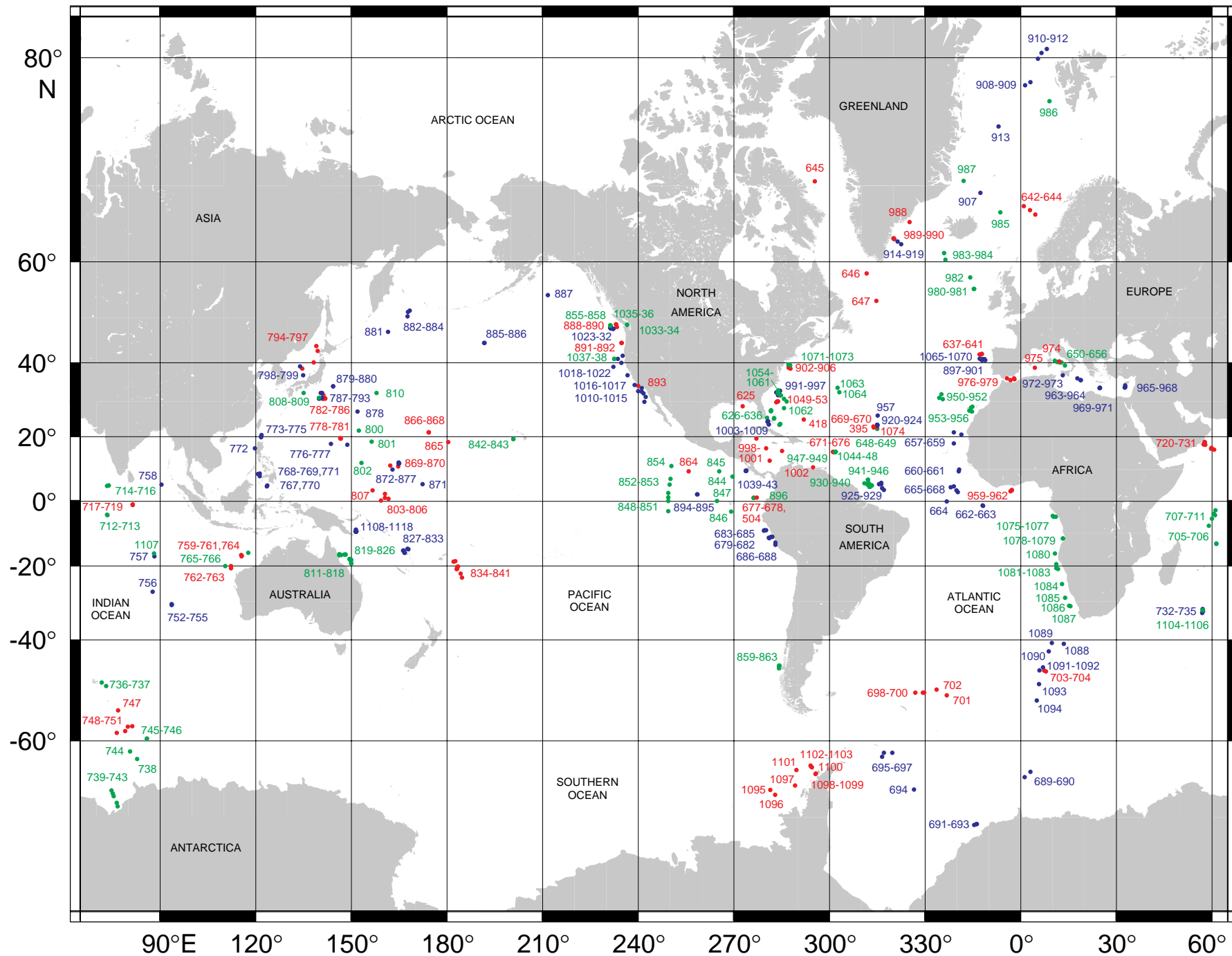
ODP Legs 100-180, Sites 625-1118
