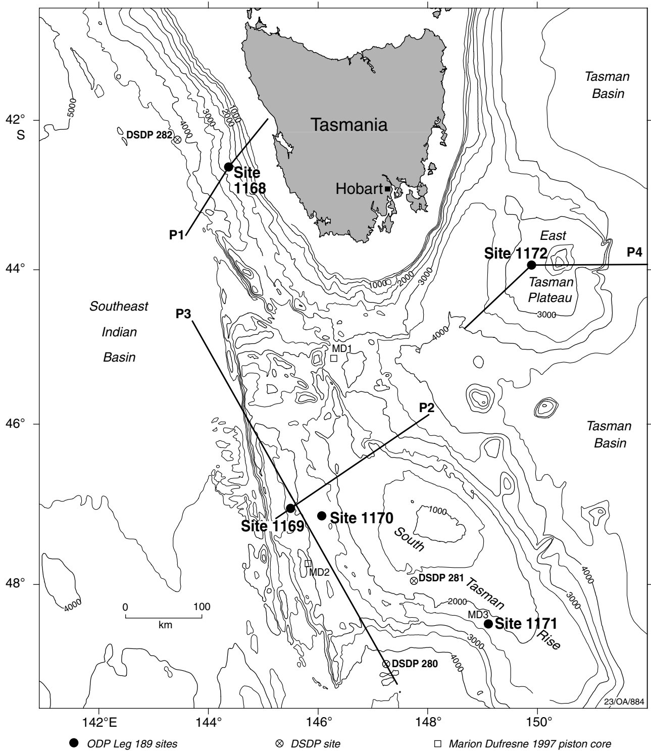
ODP Leg 189 Site Map
