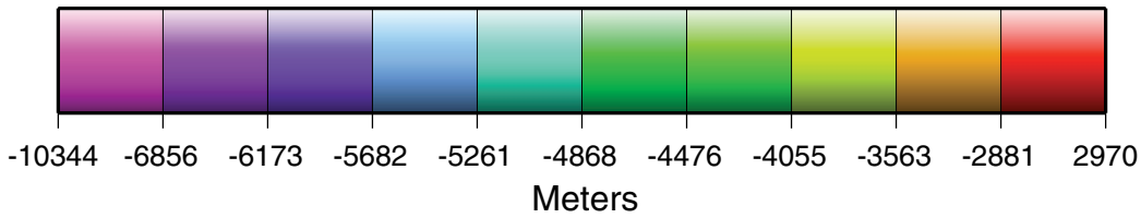
ODP Leg 191 Site Map
