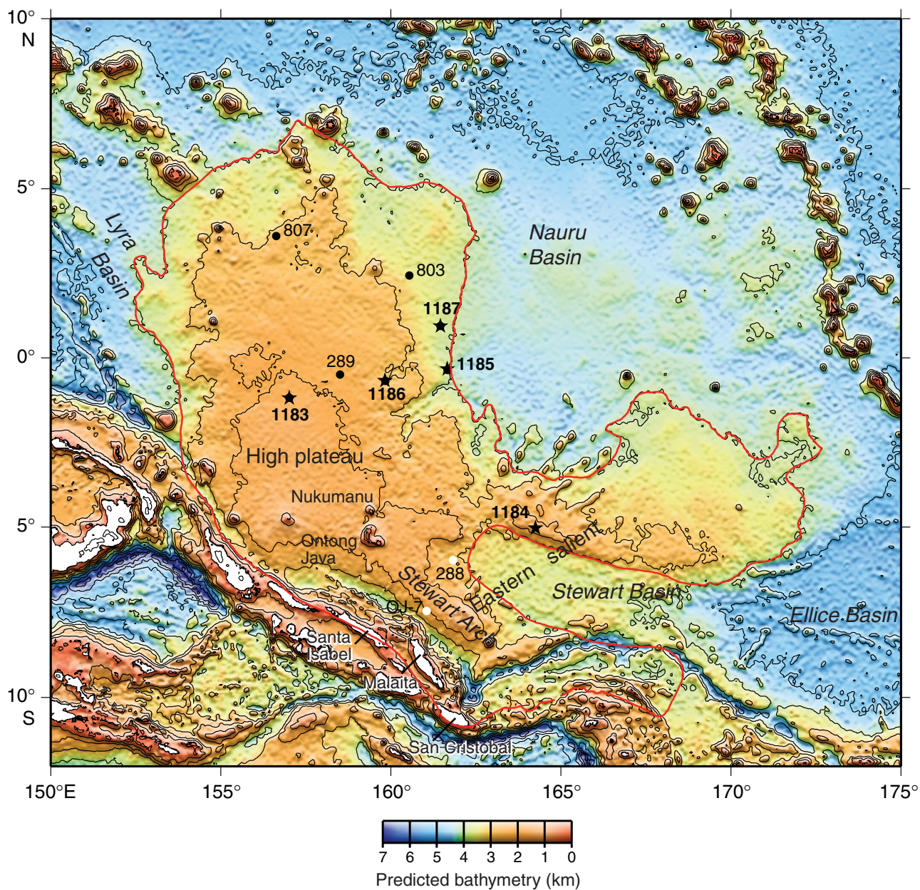
ODP Leg 192 Site Map
