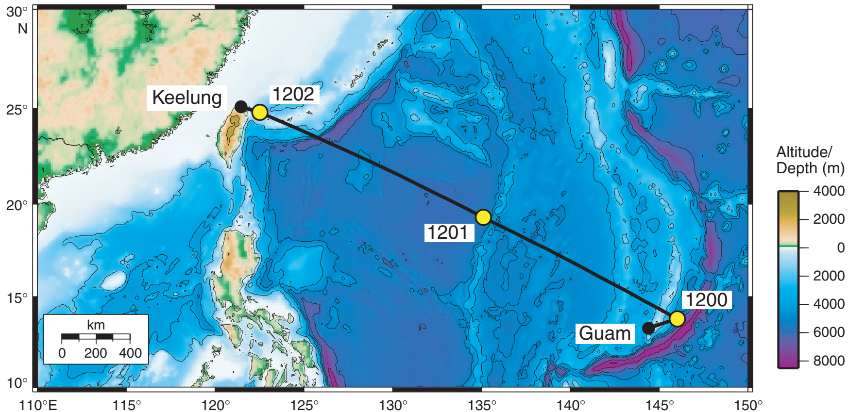
ODP Leg 195 Site Map
