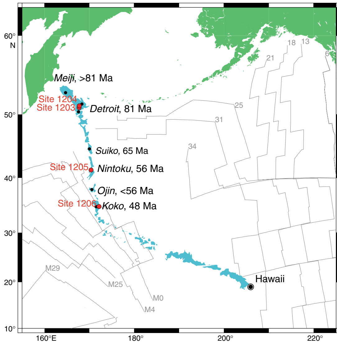
ODP Leg 197 Site Map
