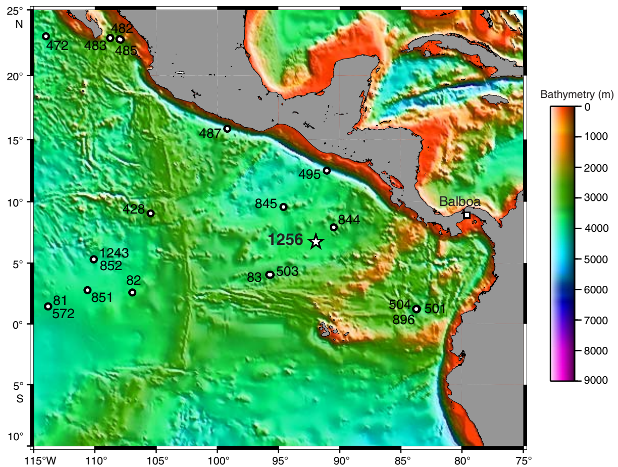
ODP Leg 206 Site Map
