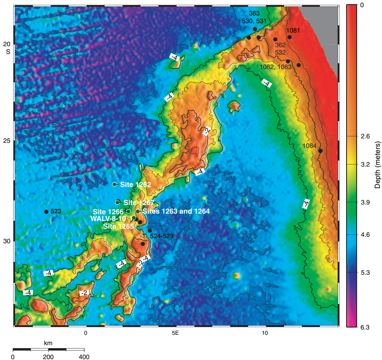
ODP Leg 208 Site Map
